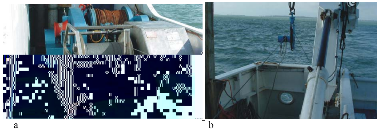
Fig. 6 : Treuil avec son câble électro-porteur (a) et sa poulie compteuse (b)
